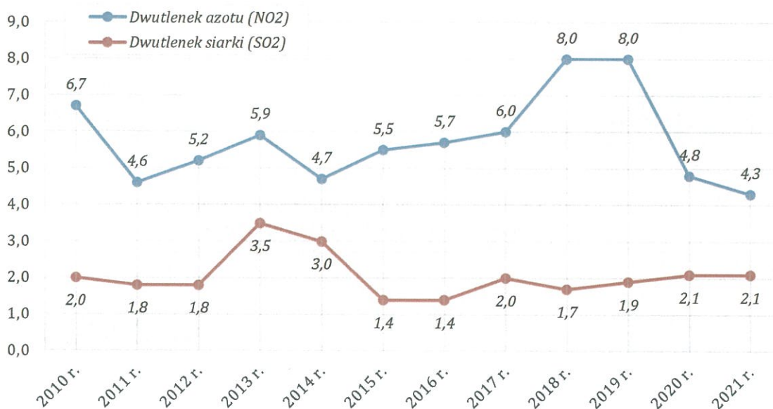
Wykres 8. Wyniki pomiarów stężeń NO 2 i SO 2 w latach 2010-2021 na stacji monitoringowej GIOŚ zlokalizowanej w m. Smolary Bytnickie [stężenia średnie roczne - \mu\text{g}/\text{m}^3 ]
